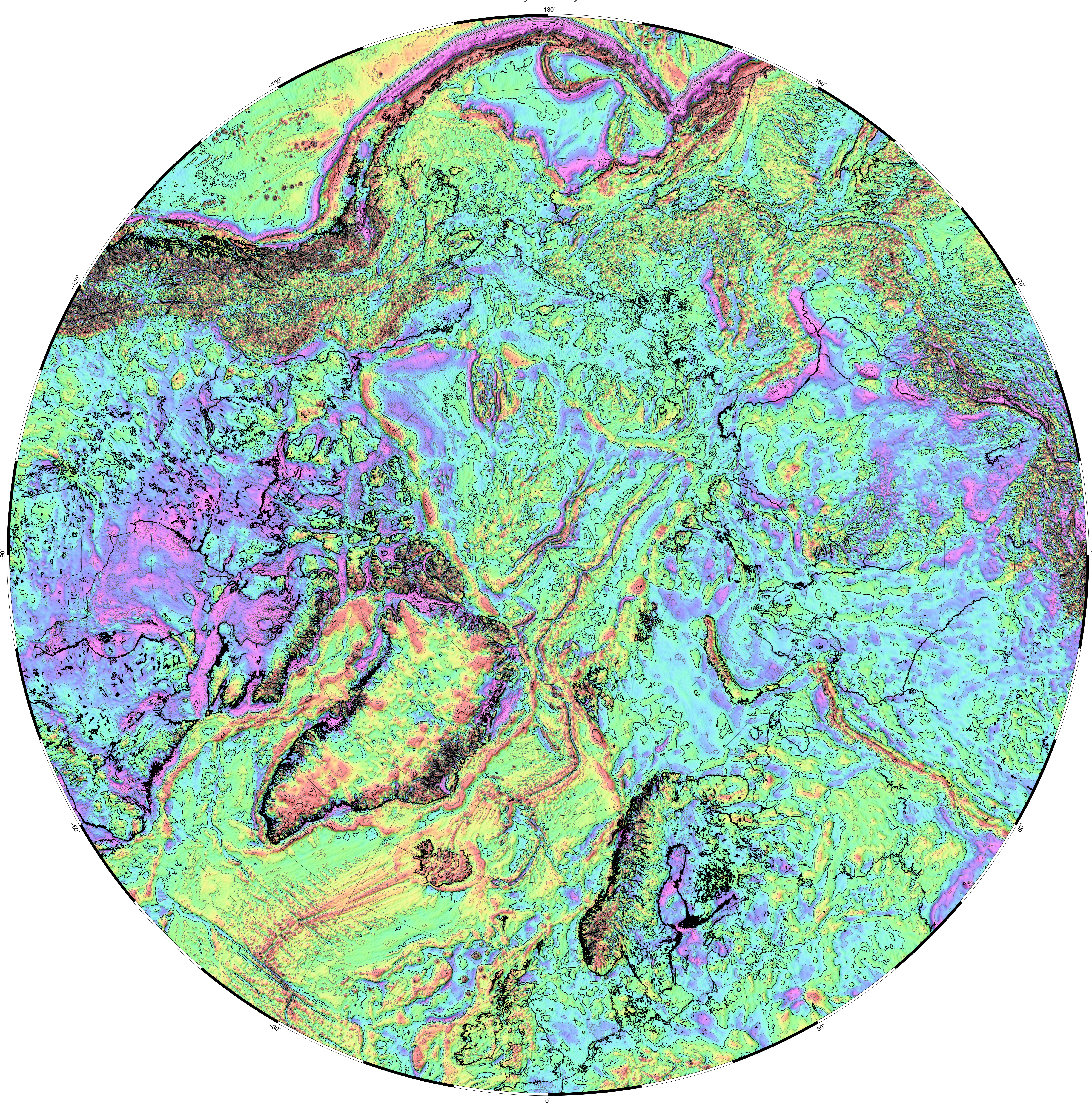
Gravity Anomaly V26
